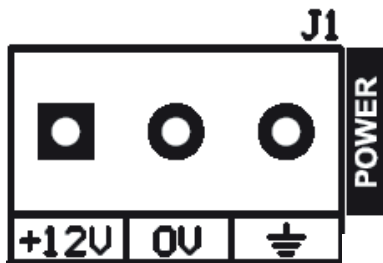
Figura 2. Conexión alimentación módulo principal.
