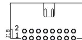
Figura 12. Conexión expansión E/S.
