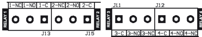
Figura 9. Conexionado salidas a relé.
