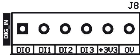
Figura 4. Conexión de entradas digitales.
